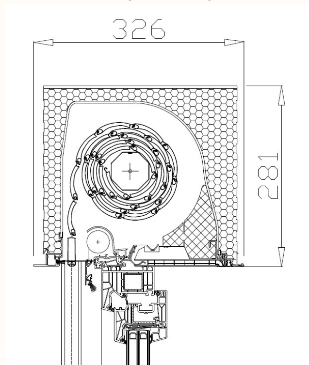
Przekrój pionowy
